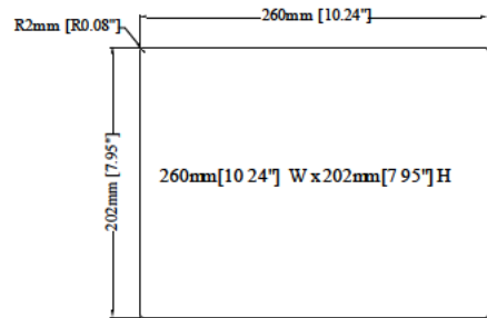
Cutout Dimensions
